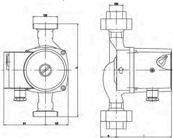
Esquema dimensional
